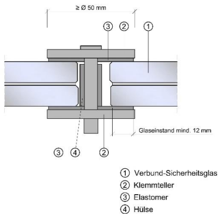
Abbildung 4: Querschnitt Tellerhalter
