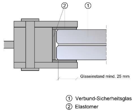
Abbildung 5: Querschnitt Randklemmhalter
